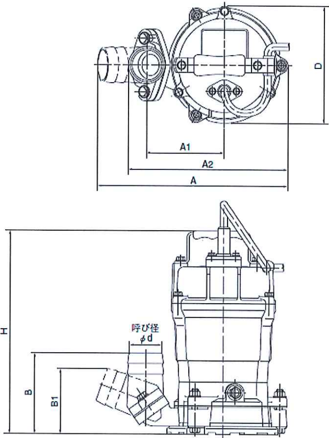
外形寸法図
